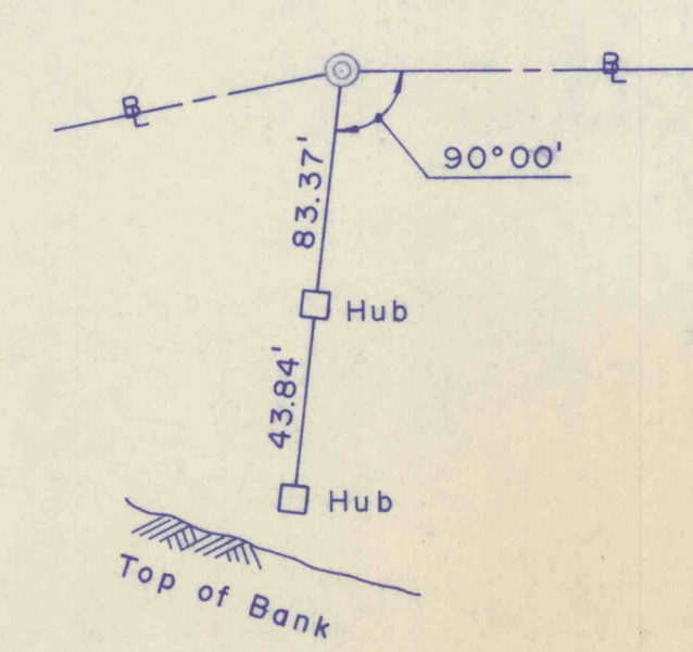
STA. 26+84.10
