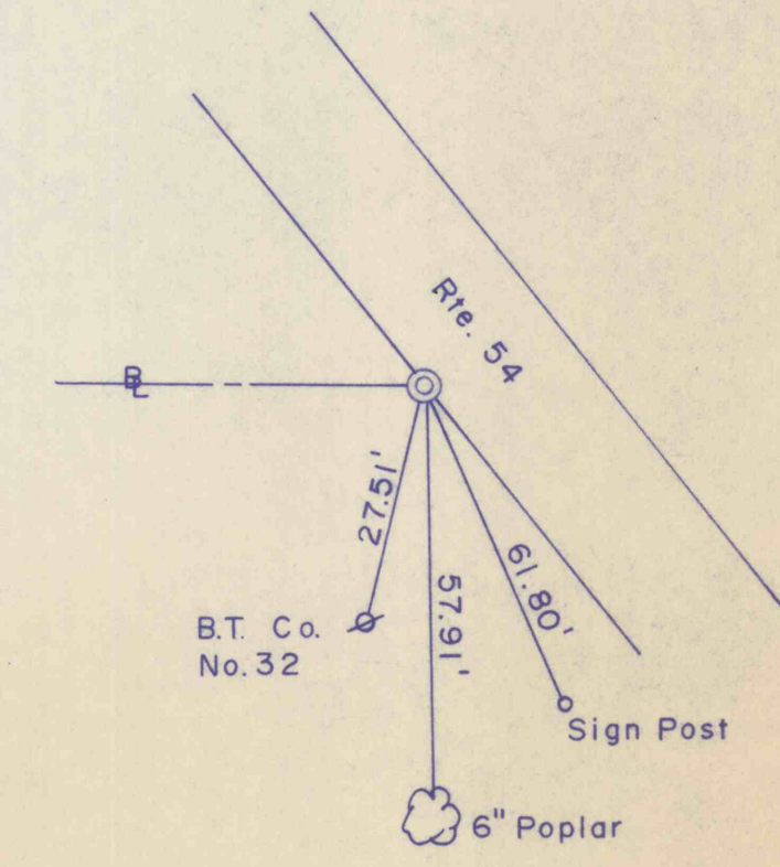
STA. 0+00
