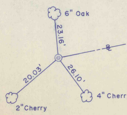
STA. 53+11.25
