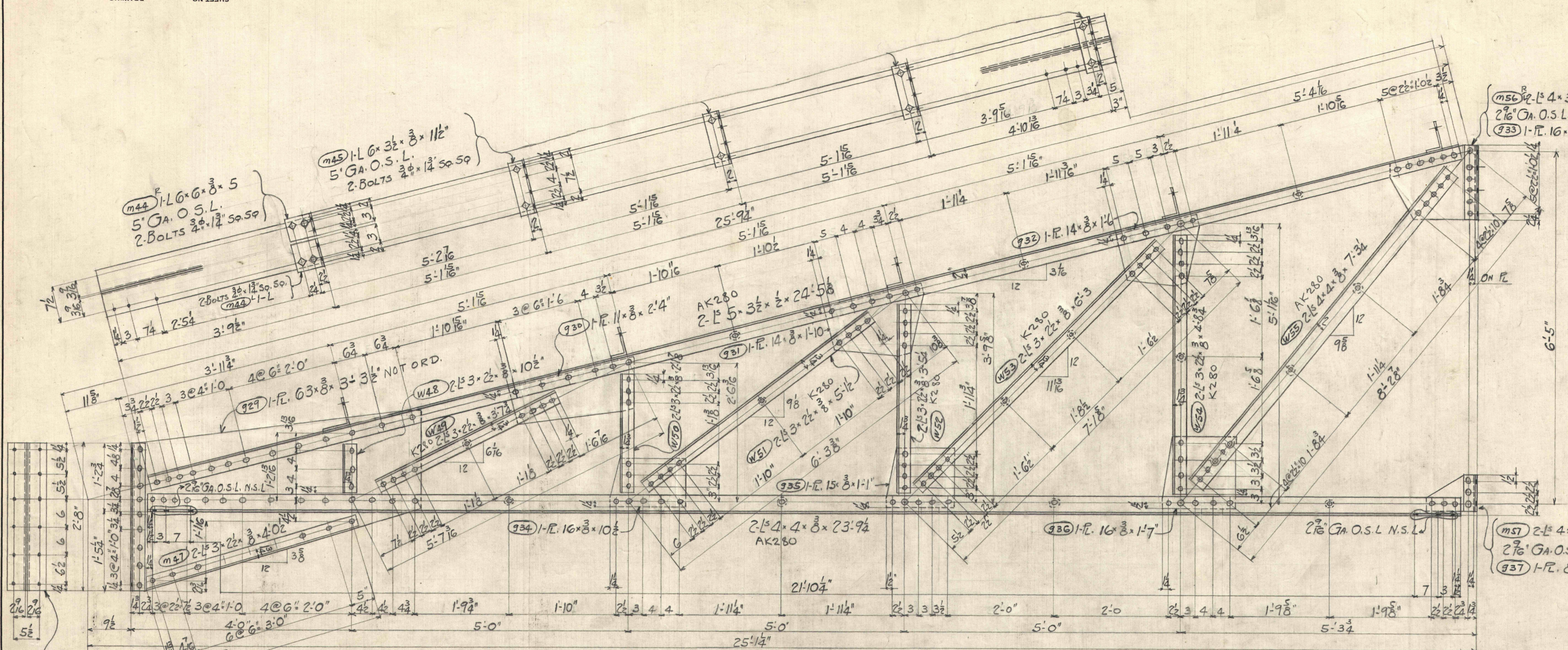
1-TRUSS T6
