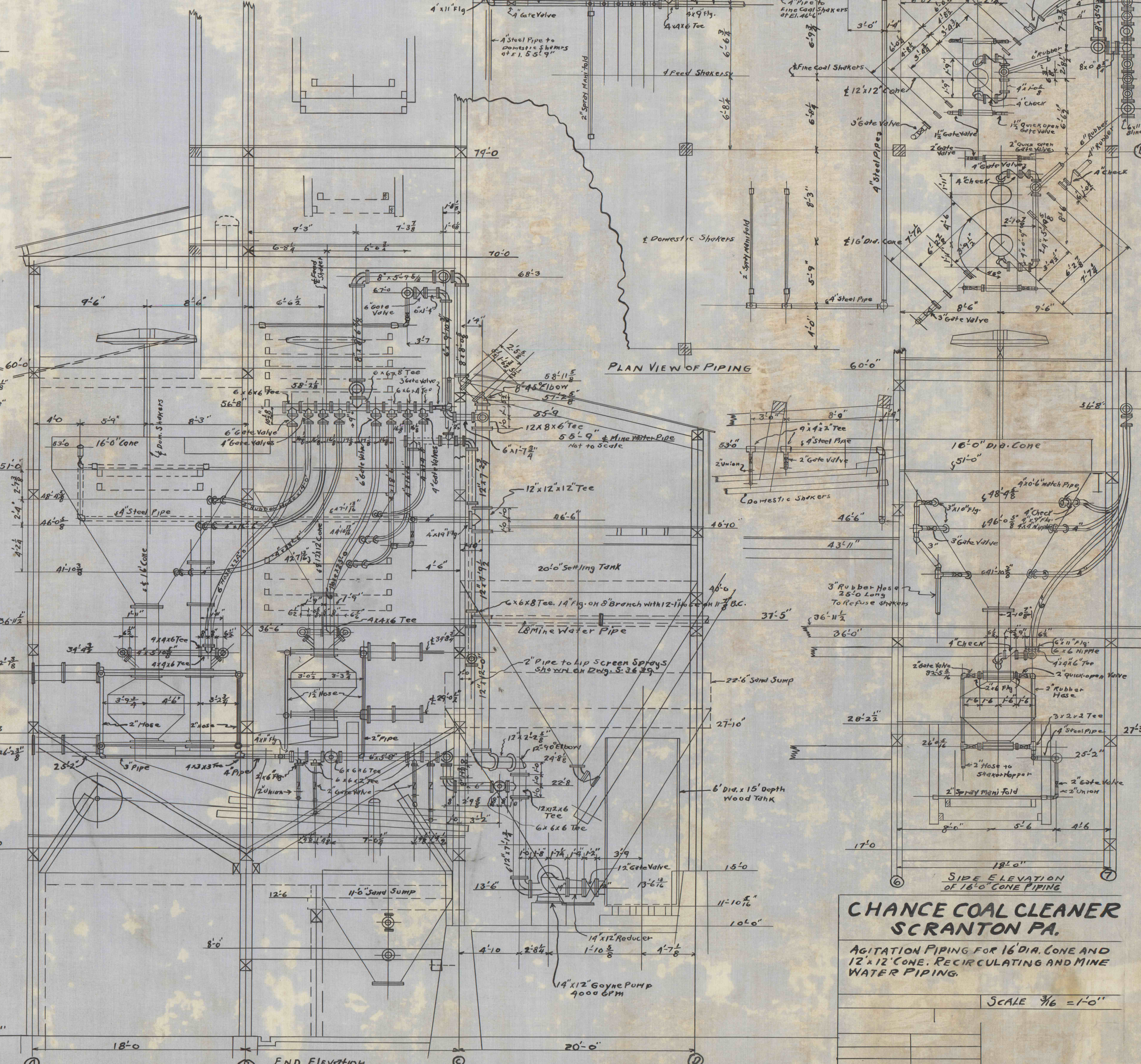
END ELEVATION
