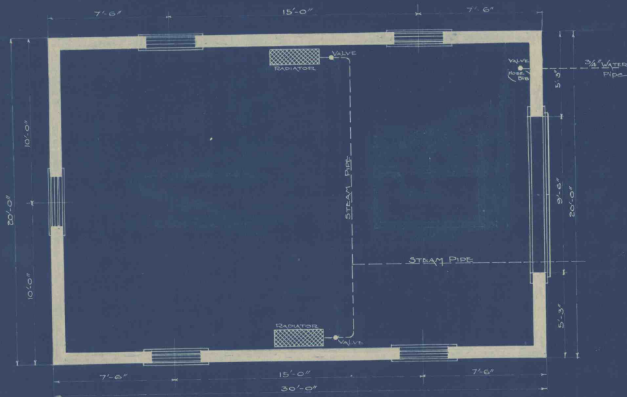
PLAN Scale: 4 Feet per inch.
