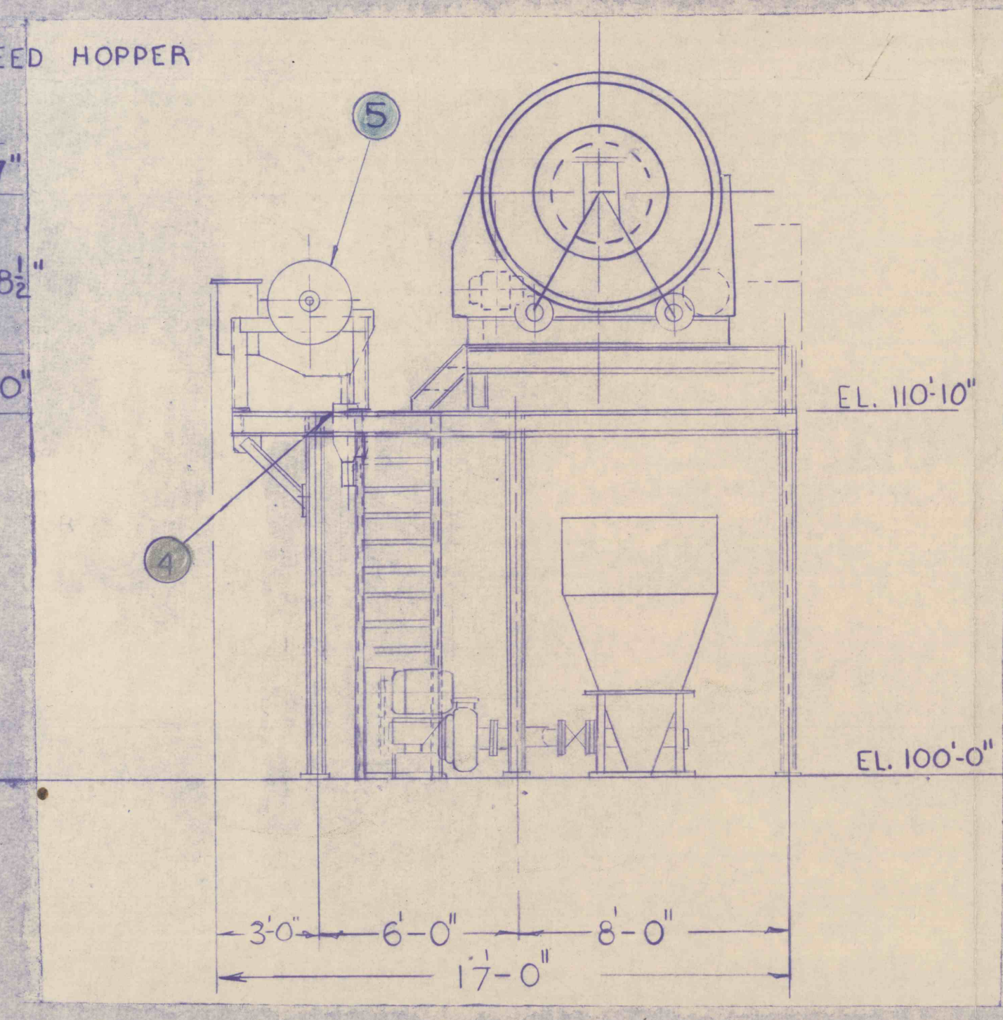
END ELEVATION
