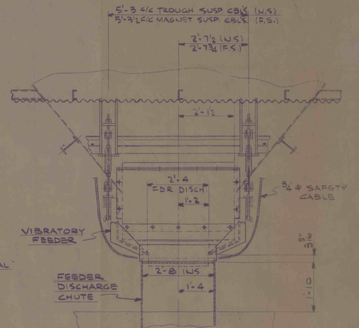
SECTION A-A
