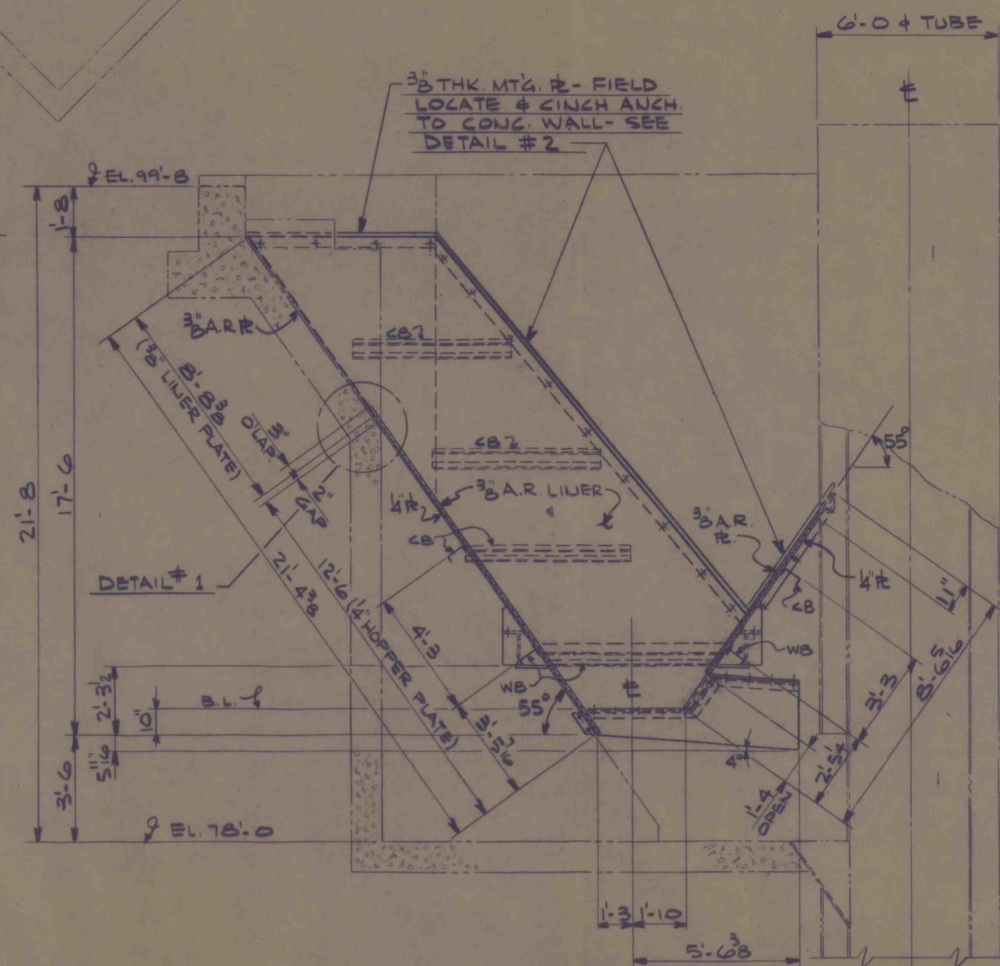
SECTION A-A
