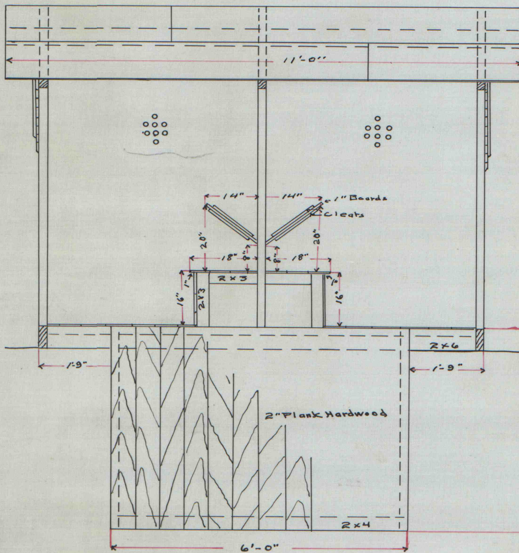
Side Elev
