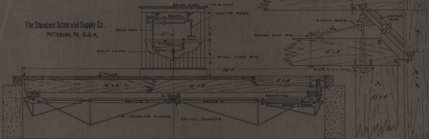
Longitudinal Section
