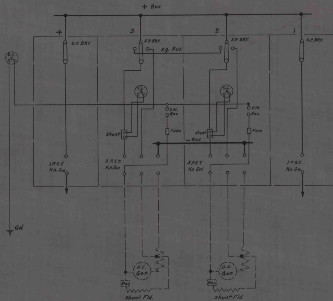
Wiring Diagram.
