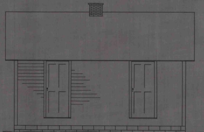
— Front Elev. —
