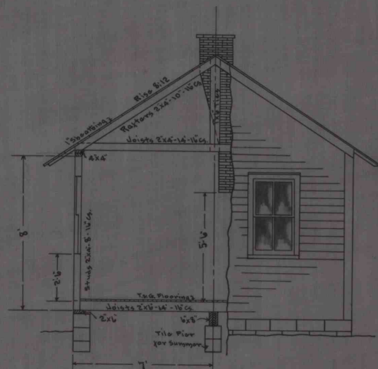
— Cross Section & Elev. —
