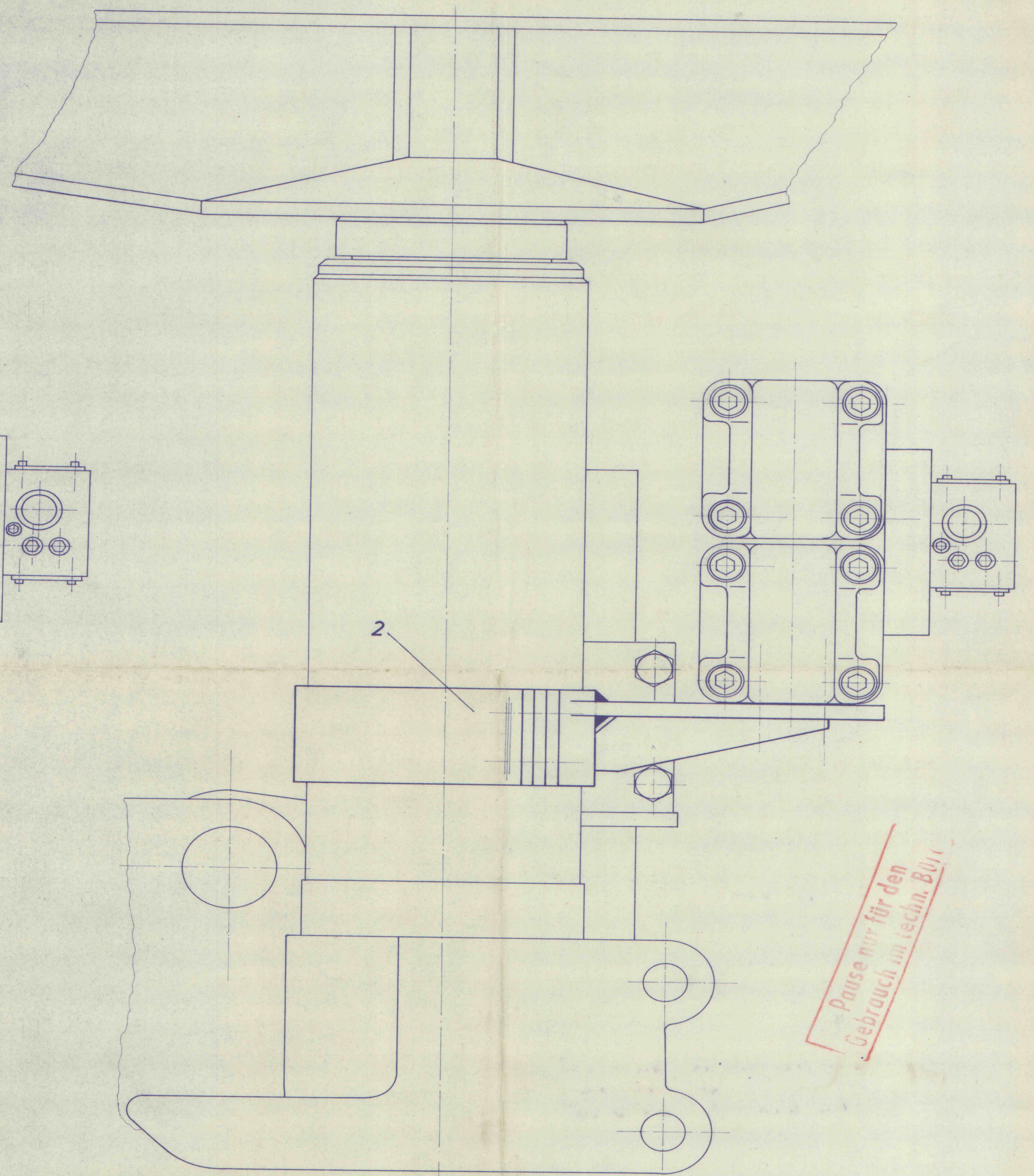
Ansicht in Richtung „B“ (siehe Blatt 1)
