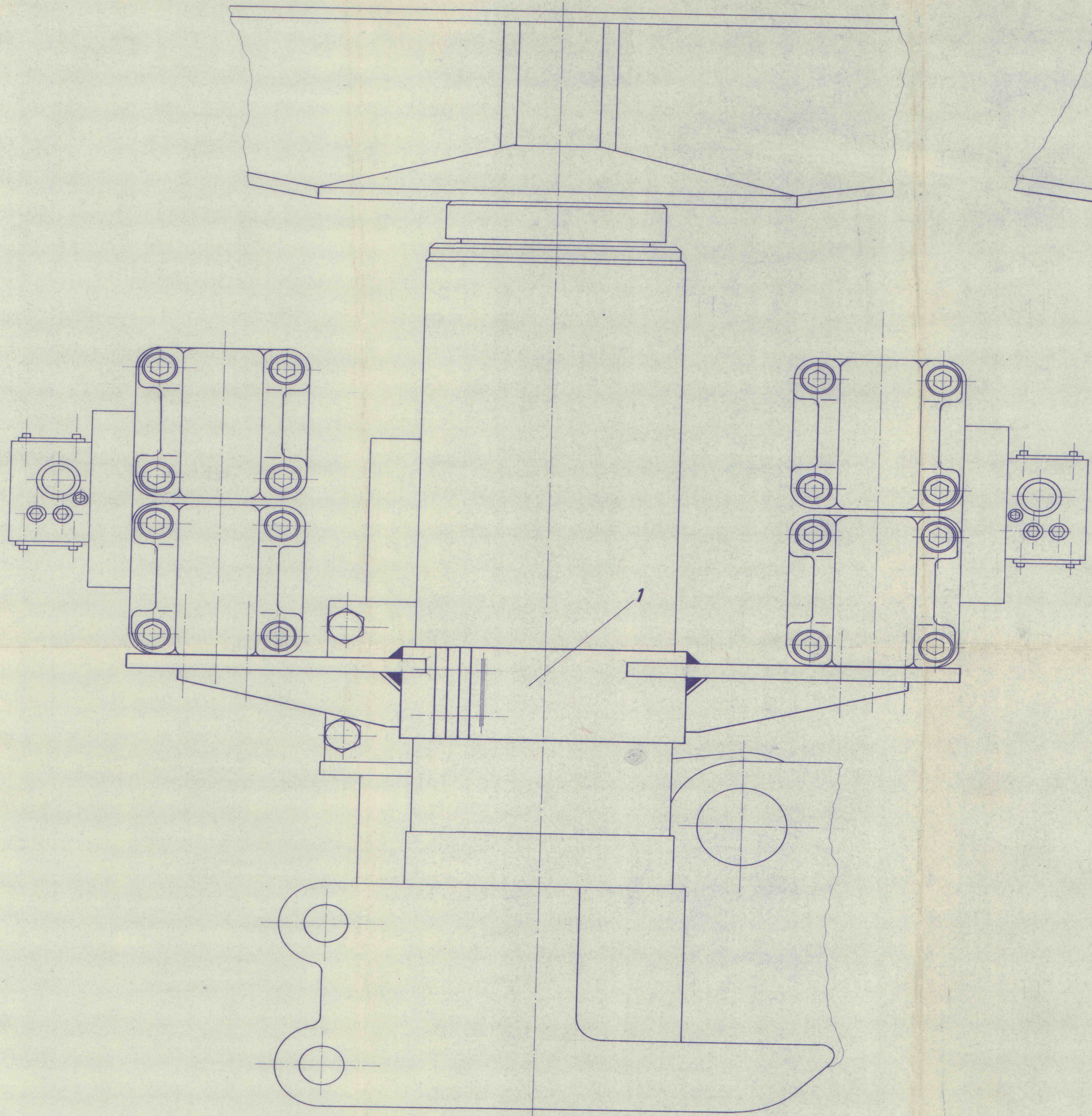
Ansicht in Richtung „A“ (siehe Blatt 1)
