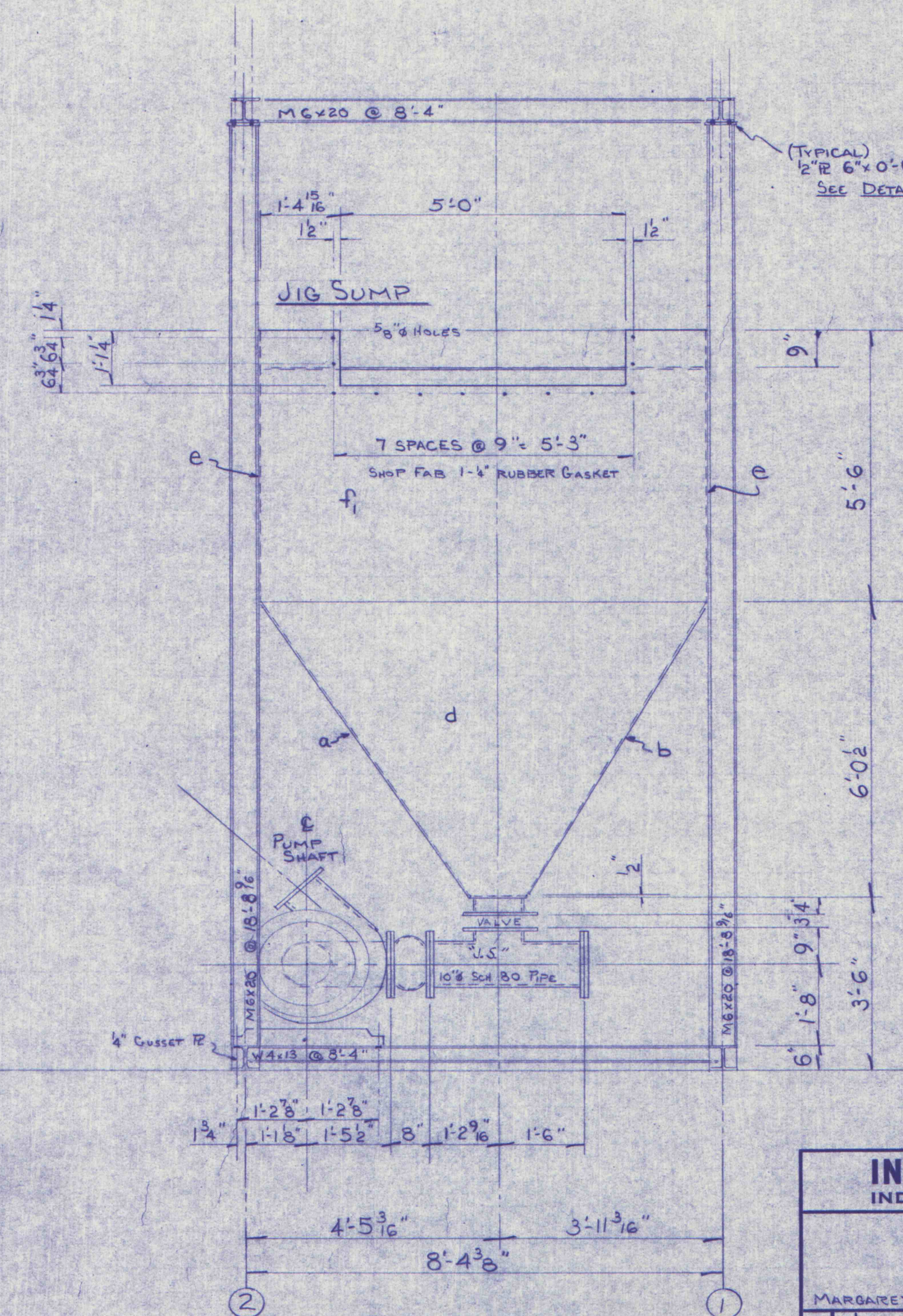
SECTION A-A
