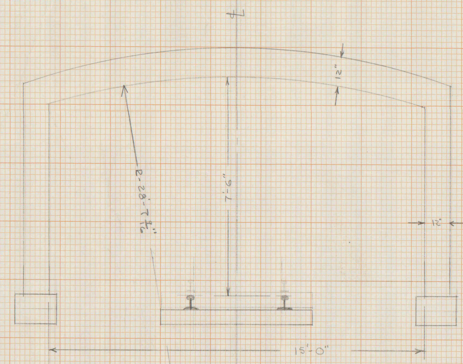
SECTION A-A.
