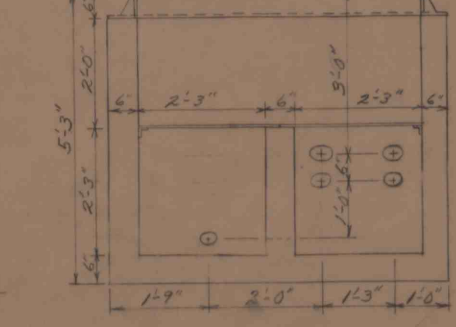
SECTION 3E-3E
