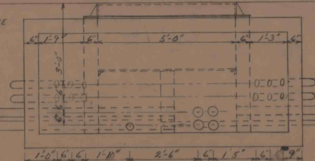
SECTION 3B-3B
