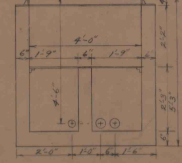
SECTION 6C-6C
