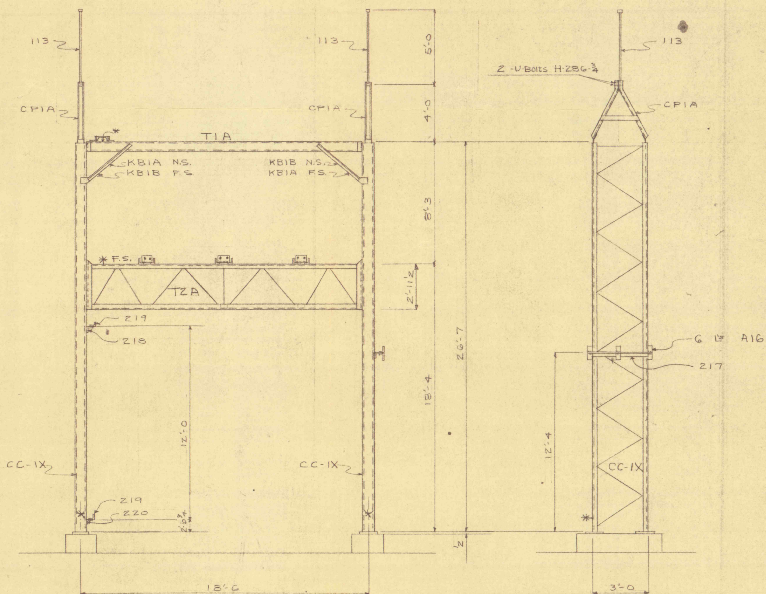
ELEVATION A-A
