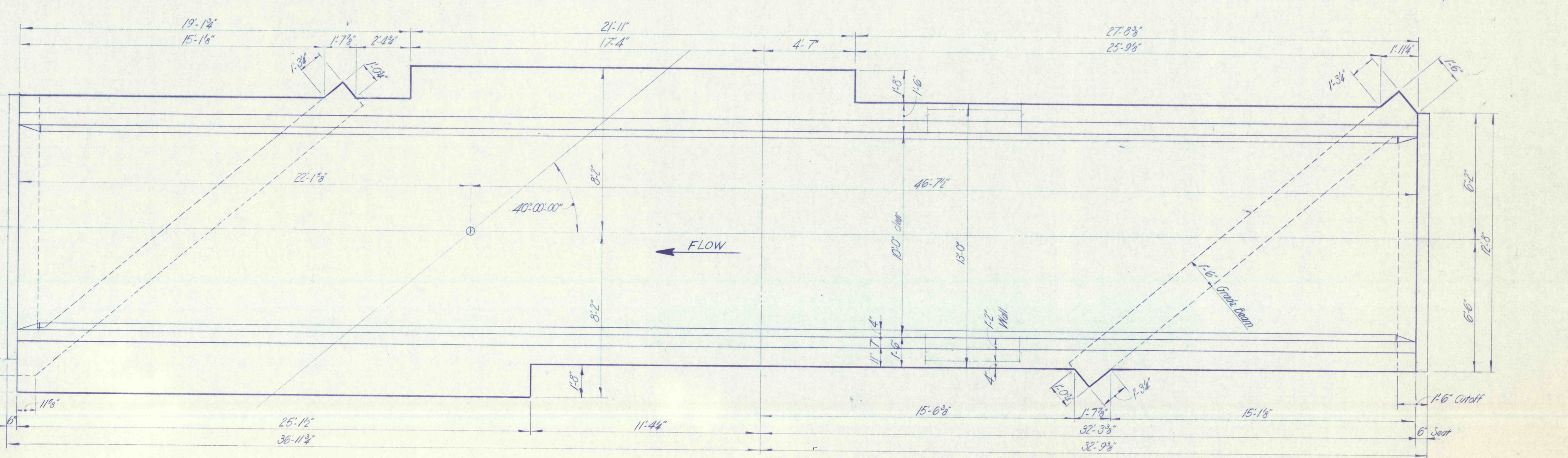
BOTTOM SLAB PLAN Scale: 3/8" = 1'-0"
