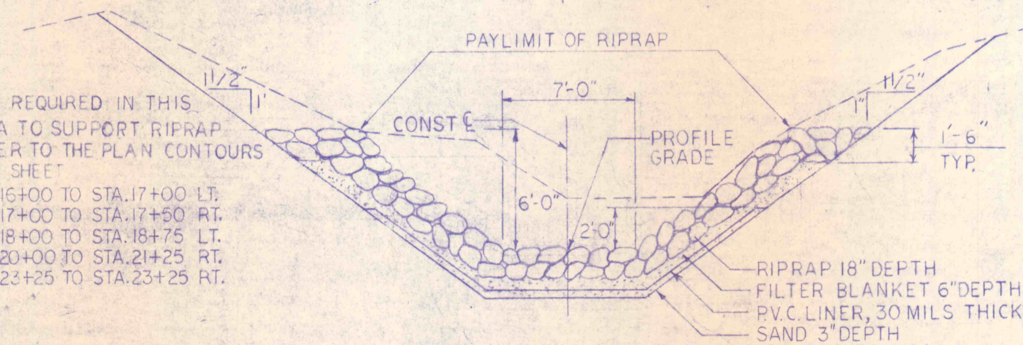
TYPICAL SECTION STA. 19+50 TO STA. 24+64 SCALE: 1"=5'
