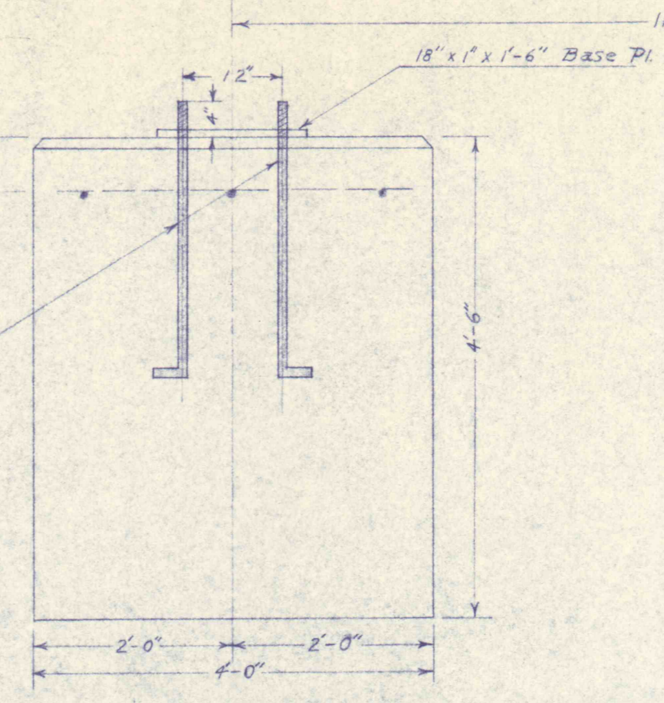
Tower Pier Y
