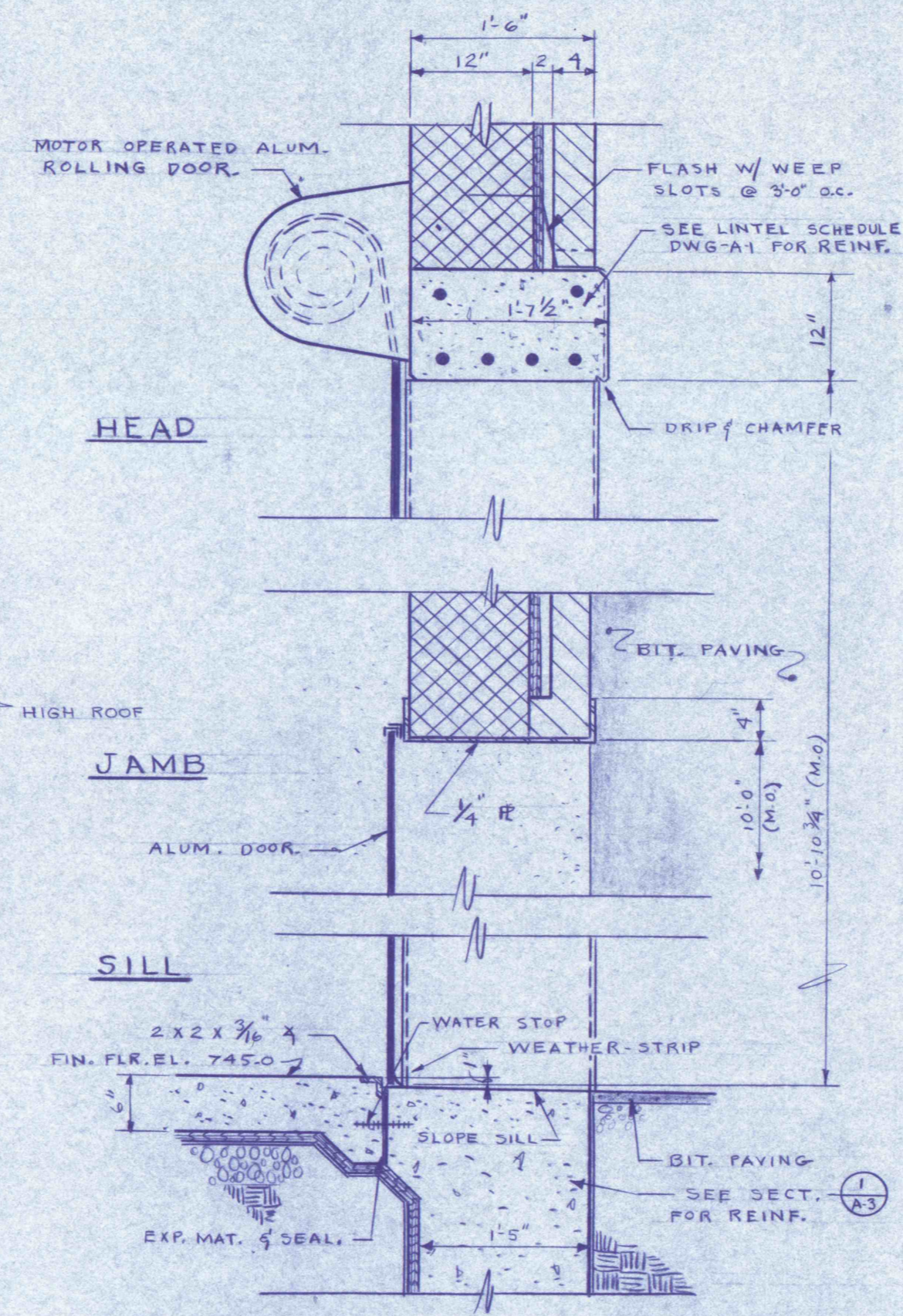
SECTION SCALE: 1/8" = 1'-0"
