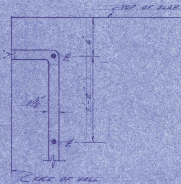
SECTION B-B SCALE: 1/2" = 1'-0"
