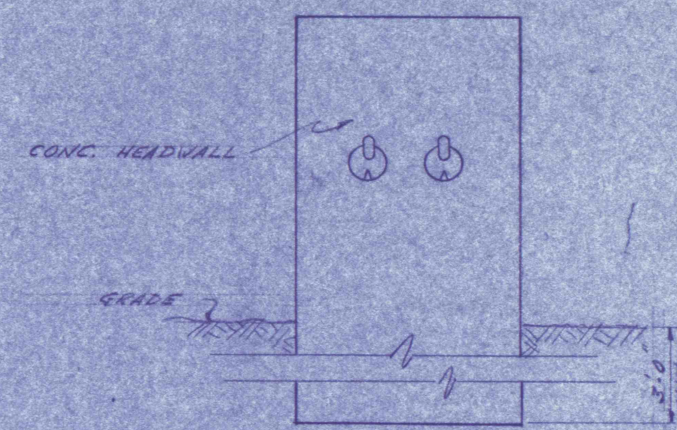
FRONT ELEV. SCALE: 1/2" = 1'-0"
