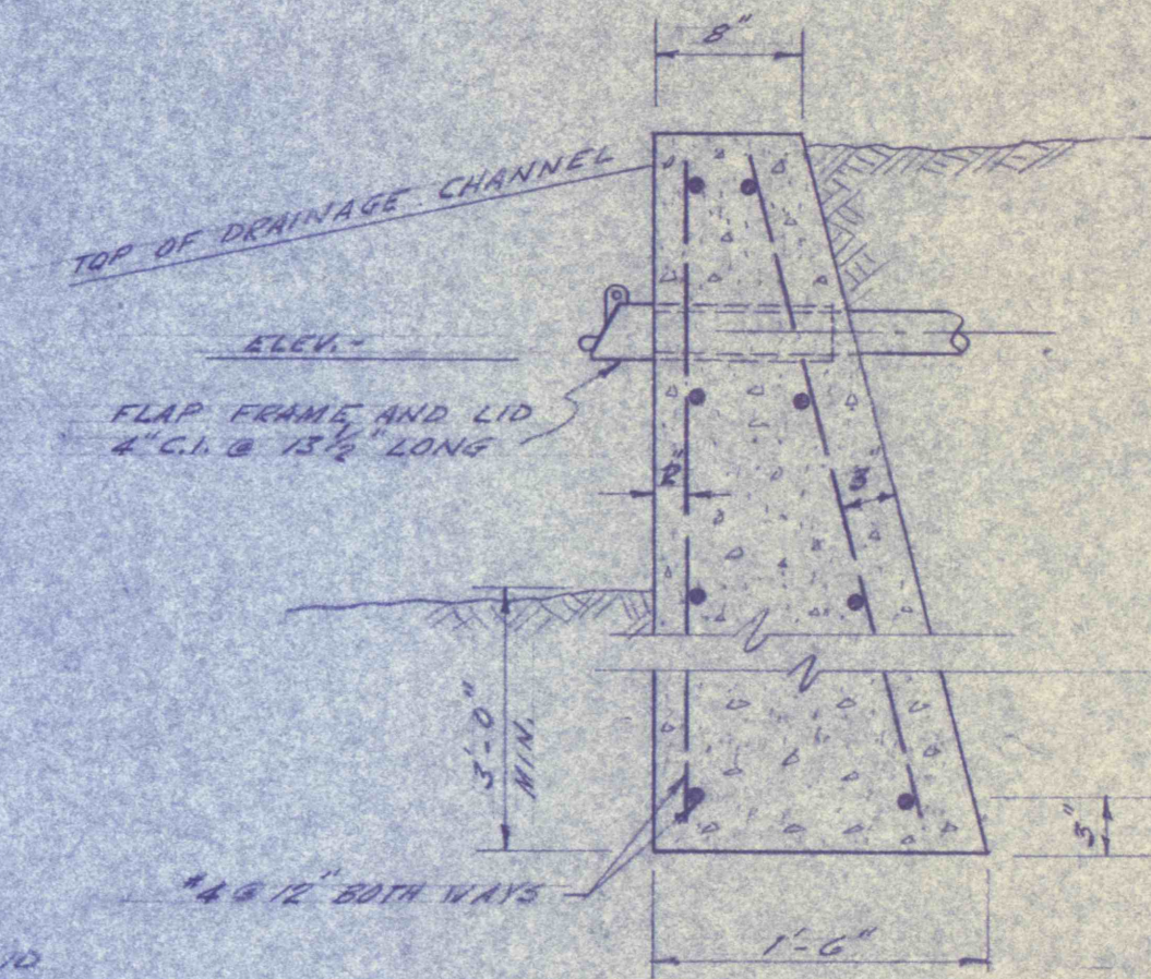
SECTION D-D SCALE: 1" = 1'-0"
