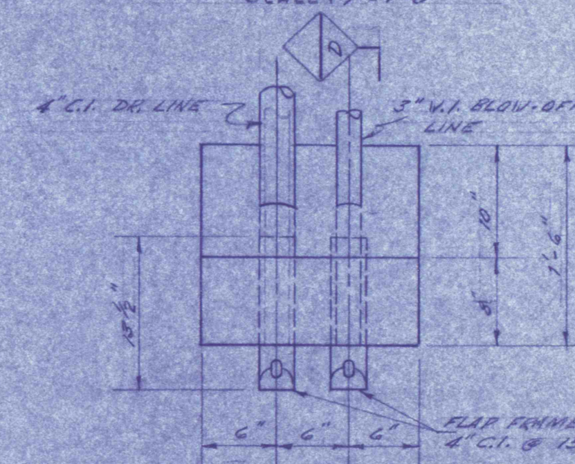
FRONT ELEV. SCALE: 1/2" = 1'-0"
