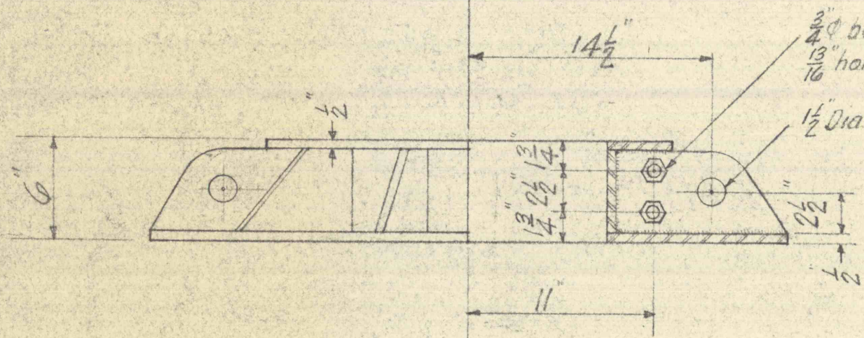
ELEVATION
