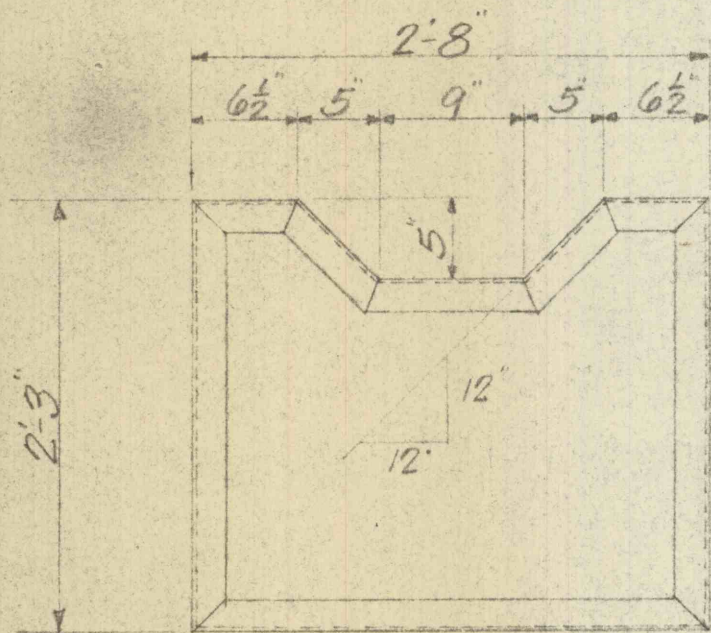
FRAME "A" 3-REQD
