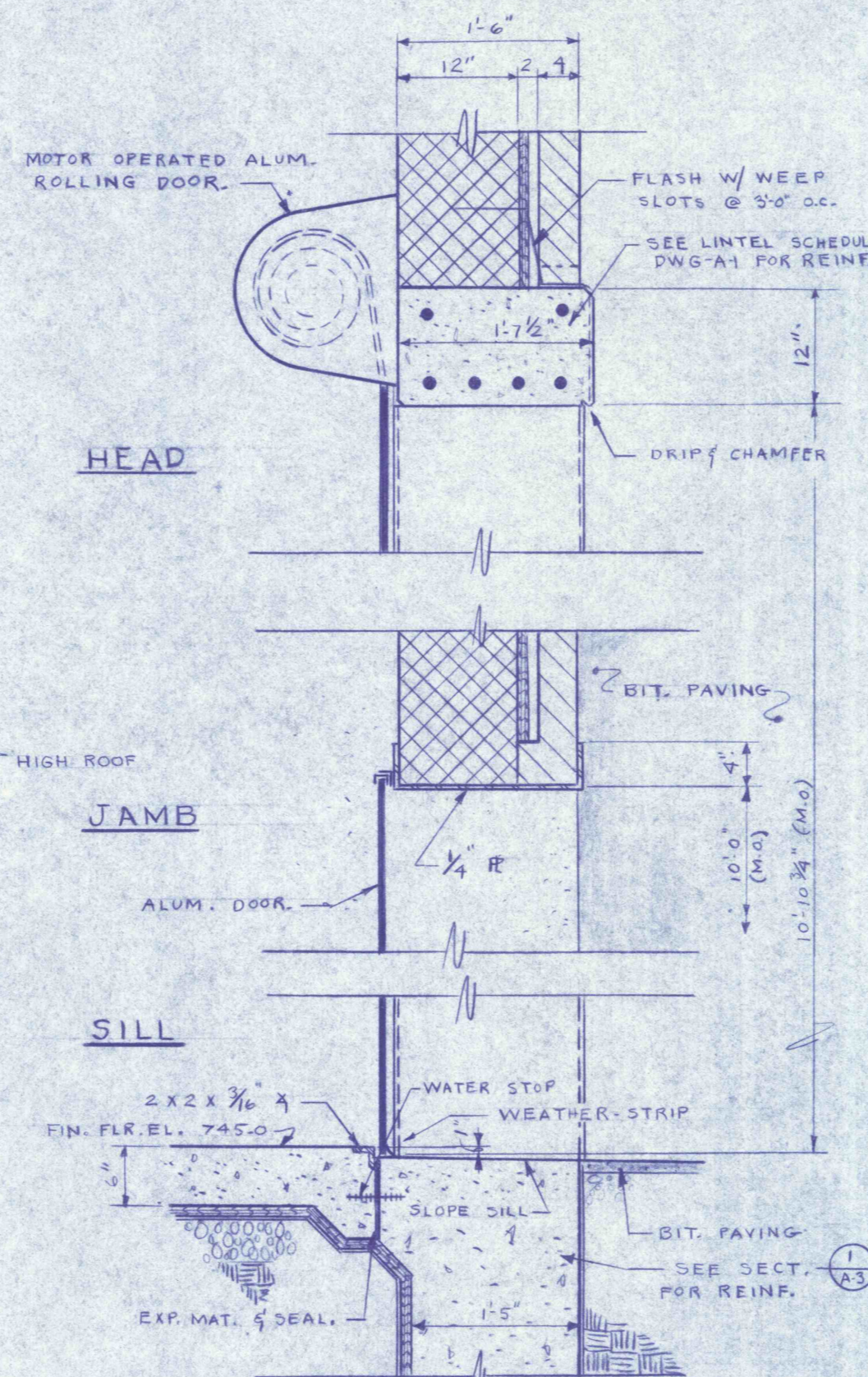
SECTION SCALE: 1/8" = 1'-0"
