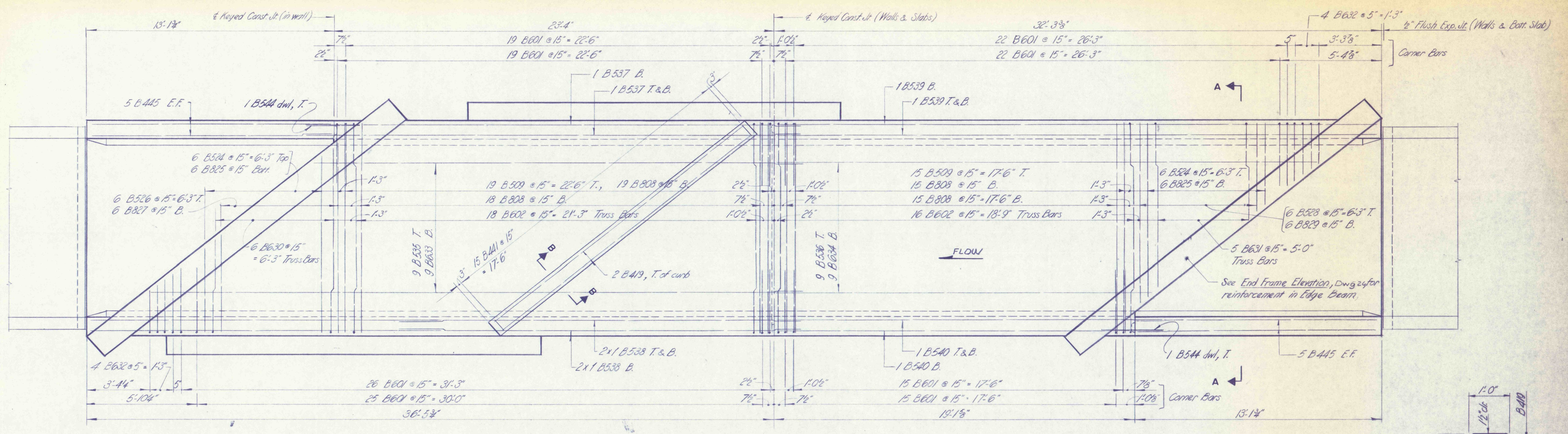
TOP SLAB PLAN Scale: 3/8" = 1'-0"
