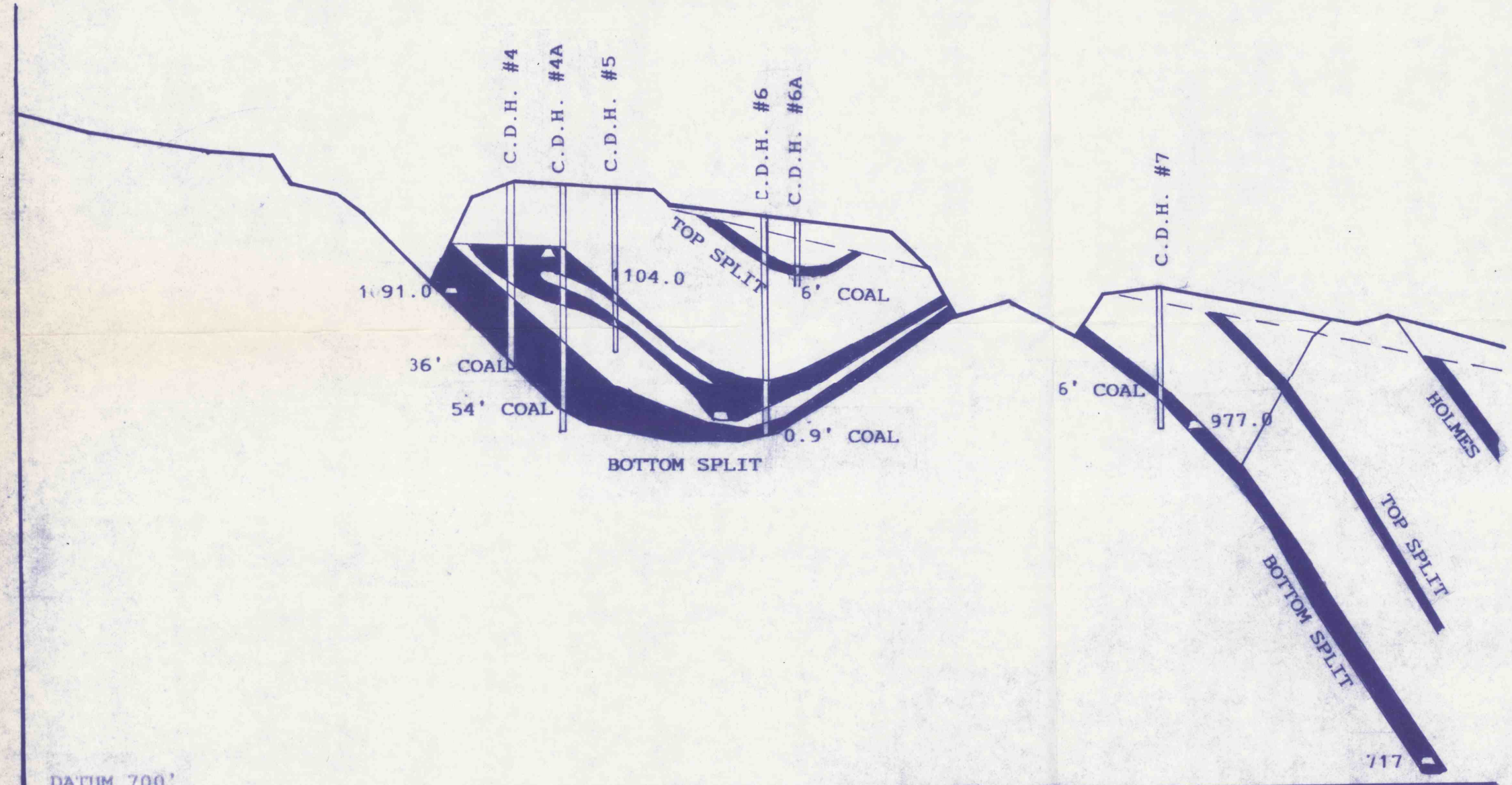
SECTION E - E
