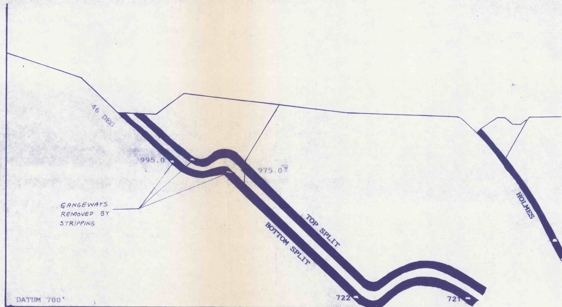
SECTION I - I
