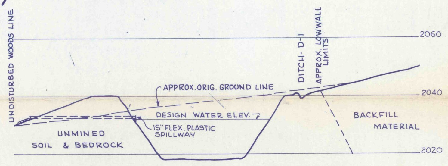
SECTION A-A' SCALE: 1" = 40' HOR. 1" = 20' VER.
