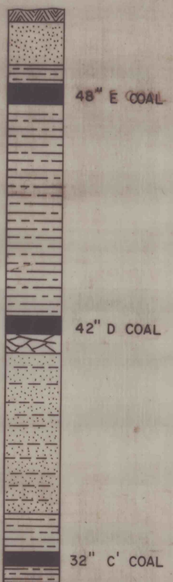
COLUMNAR SECTION SCALE: 1" = 20'
