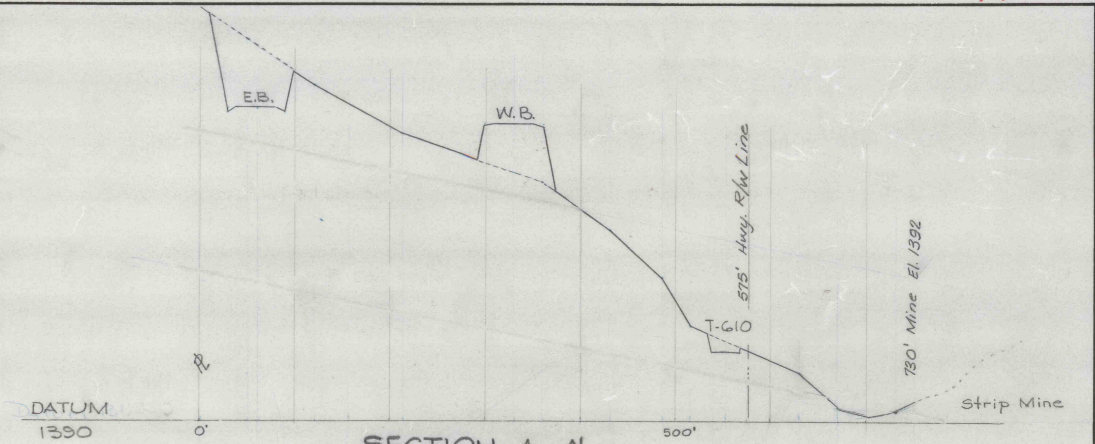
SECTION A-A'
