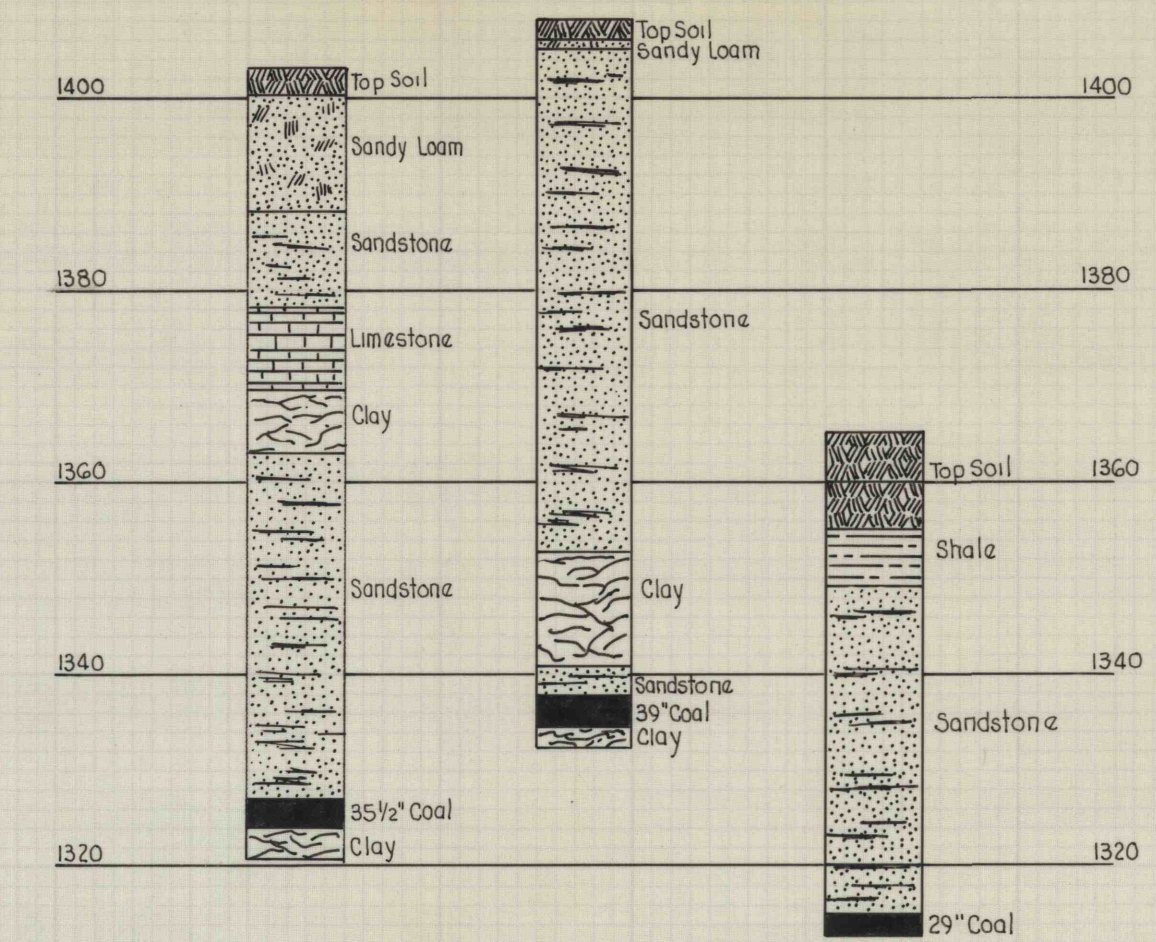
D.H. No 1 D.H. No 2 D.H. No 3 COLUMNAR SECTIONS SCALE: 1" = 20'
