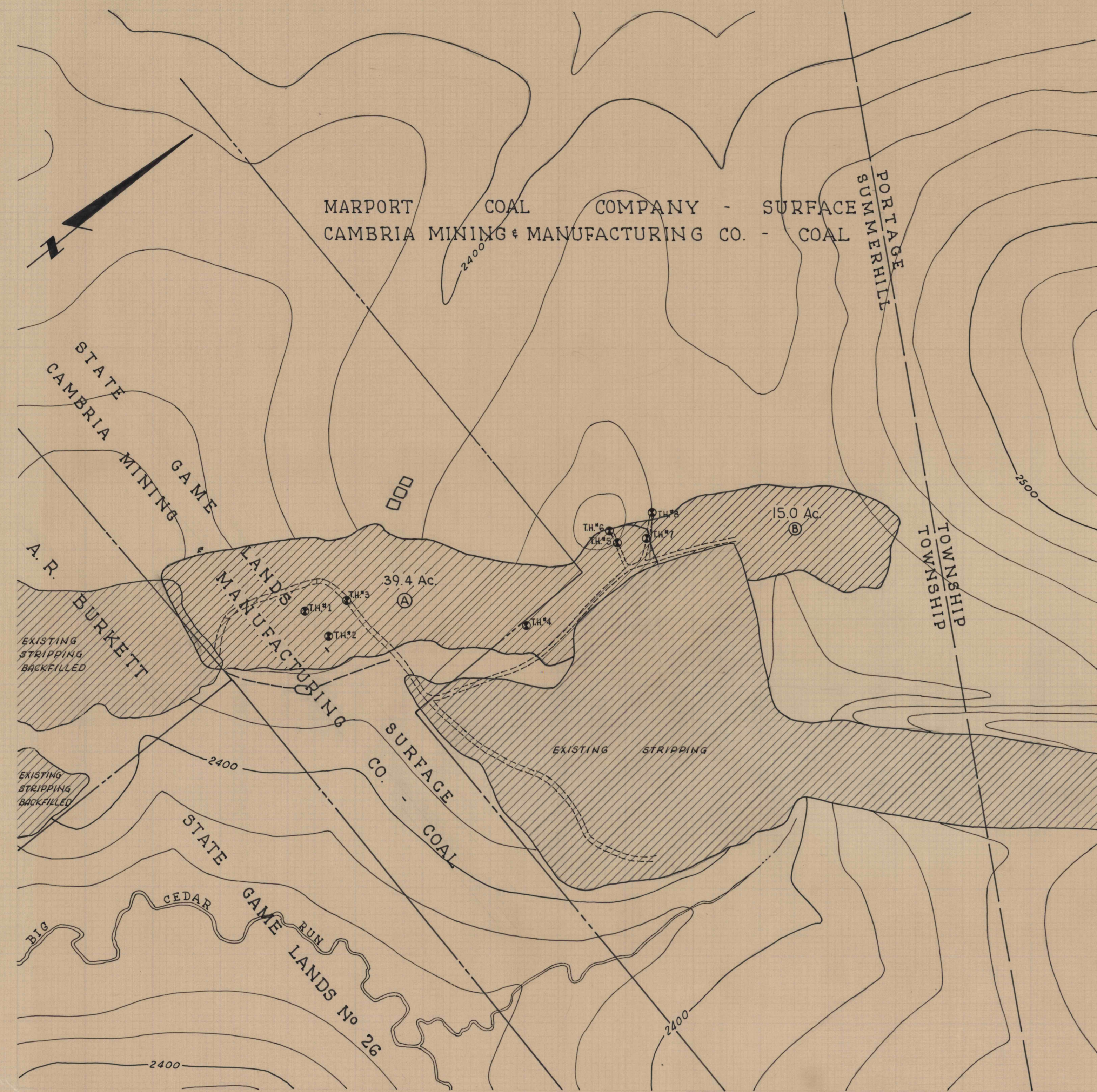
PLAN SCALE: 1" = 400'
