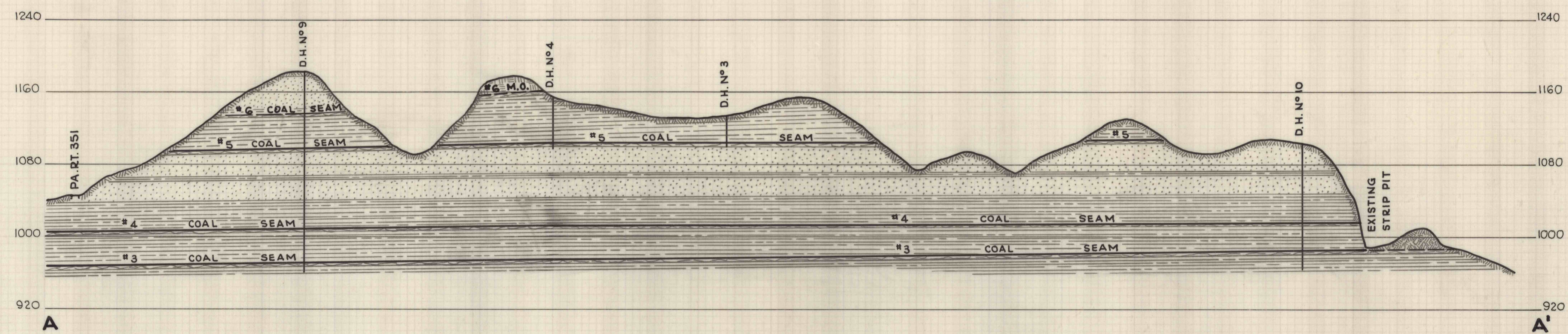
SECTION A-A'
